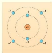
Tradiční model atomu uhlíku
