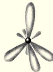
Nový model atomu uhlíku
