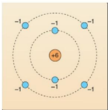
Tradiční model atomu uhlíku (elektrony ve valenčních sférách)
