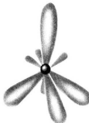
Novější model atomu uhlíku (elektrony v orbitalech - oblastech nejčastějšího výskytu)
